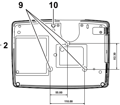
底面図
